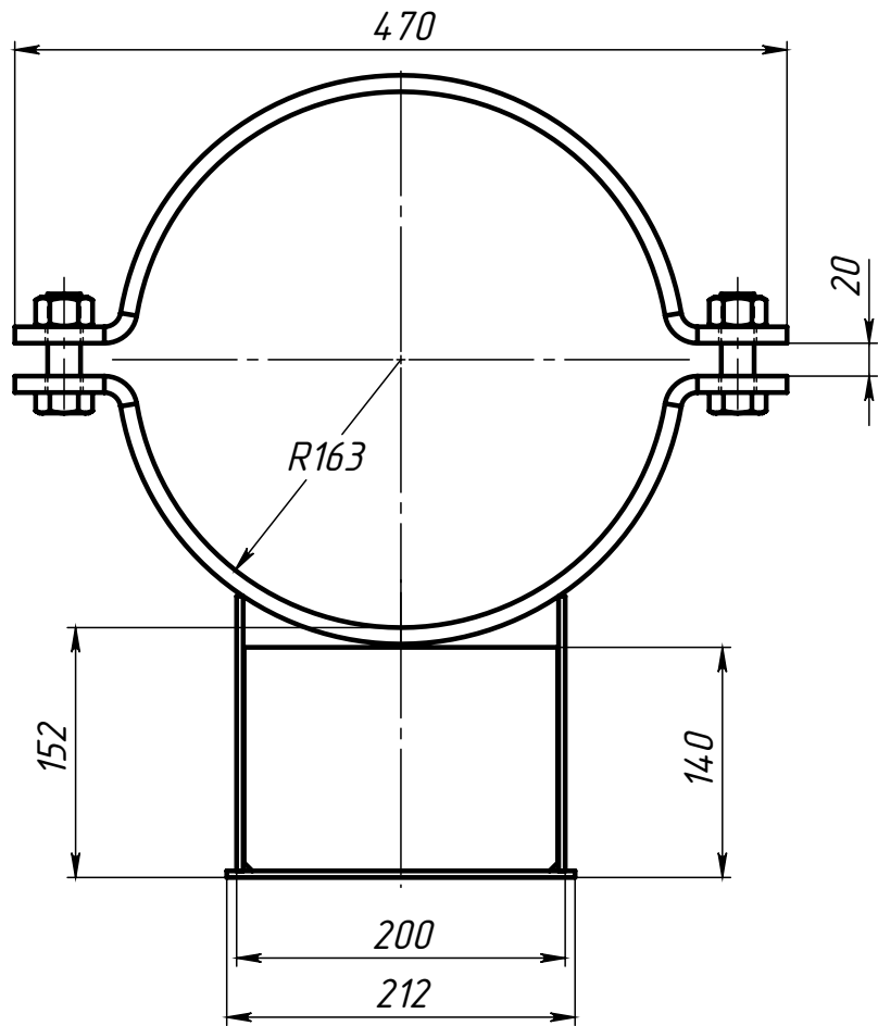
Поз.4 (Полухомут)
