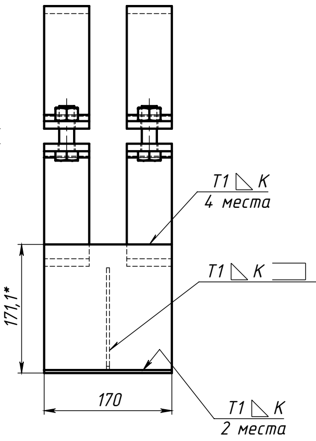
Поз.3 (Ребро среднее)
